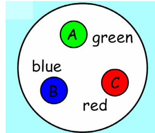
”biały” hadron (singlet koloru)
