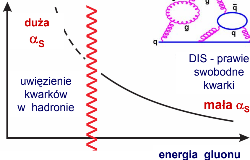
ekranowanie antyekranowanie ładunku kolorowego
