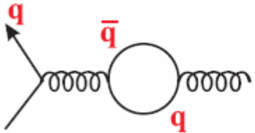
ekranowanie antyekranowanie ładunku kolorowego
