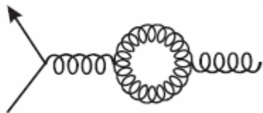
ekranowanie antyekranowanie ładunku kolorowego
